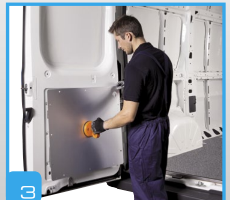
3 Door panels Paneles para puertas traseras
