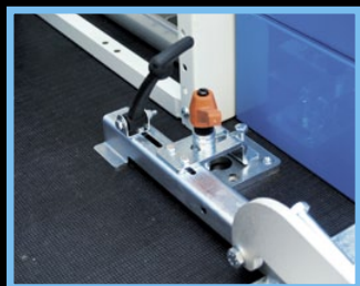
Quick fixture system left side Sistema de fijación rápida del lado izquierdo
