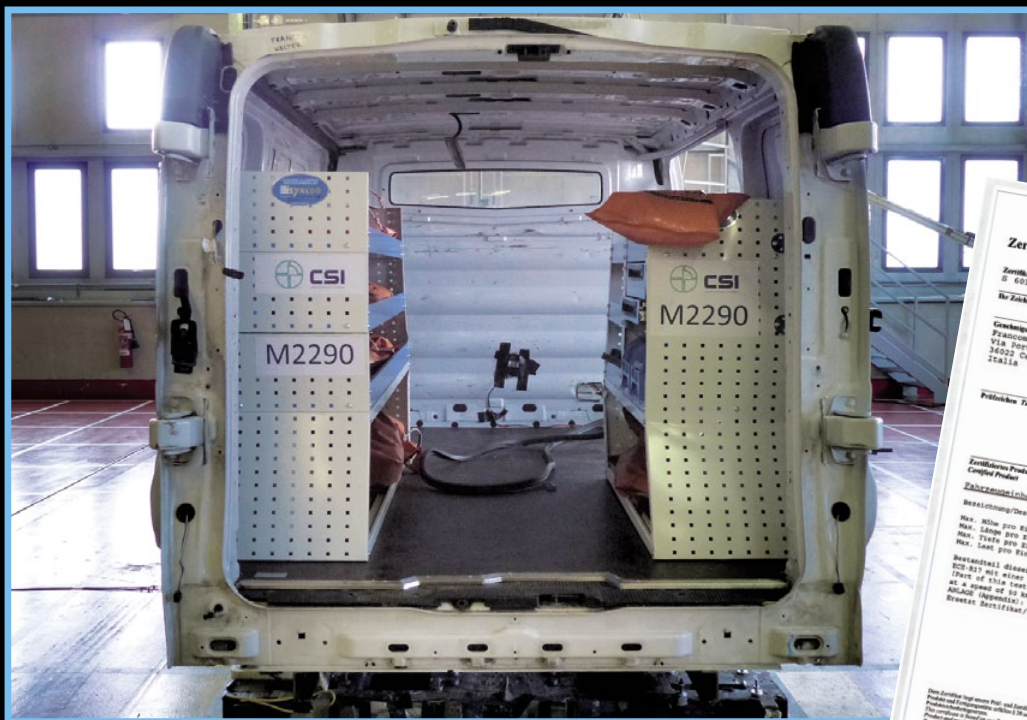
Storage units after crash test Equipamiento después de pruebas de choque
