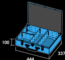
Model with dividers Modelo con divisores
